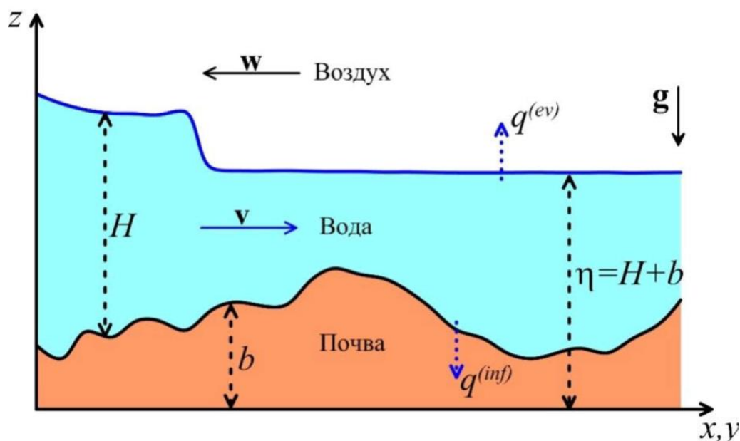
Рис. 5. Схема, поясняющая обозначения математической модели.
