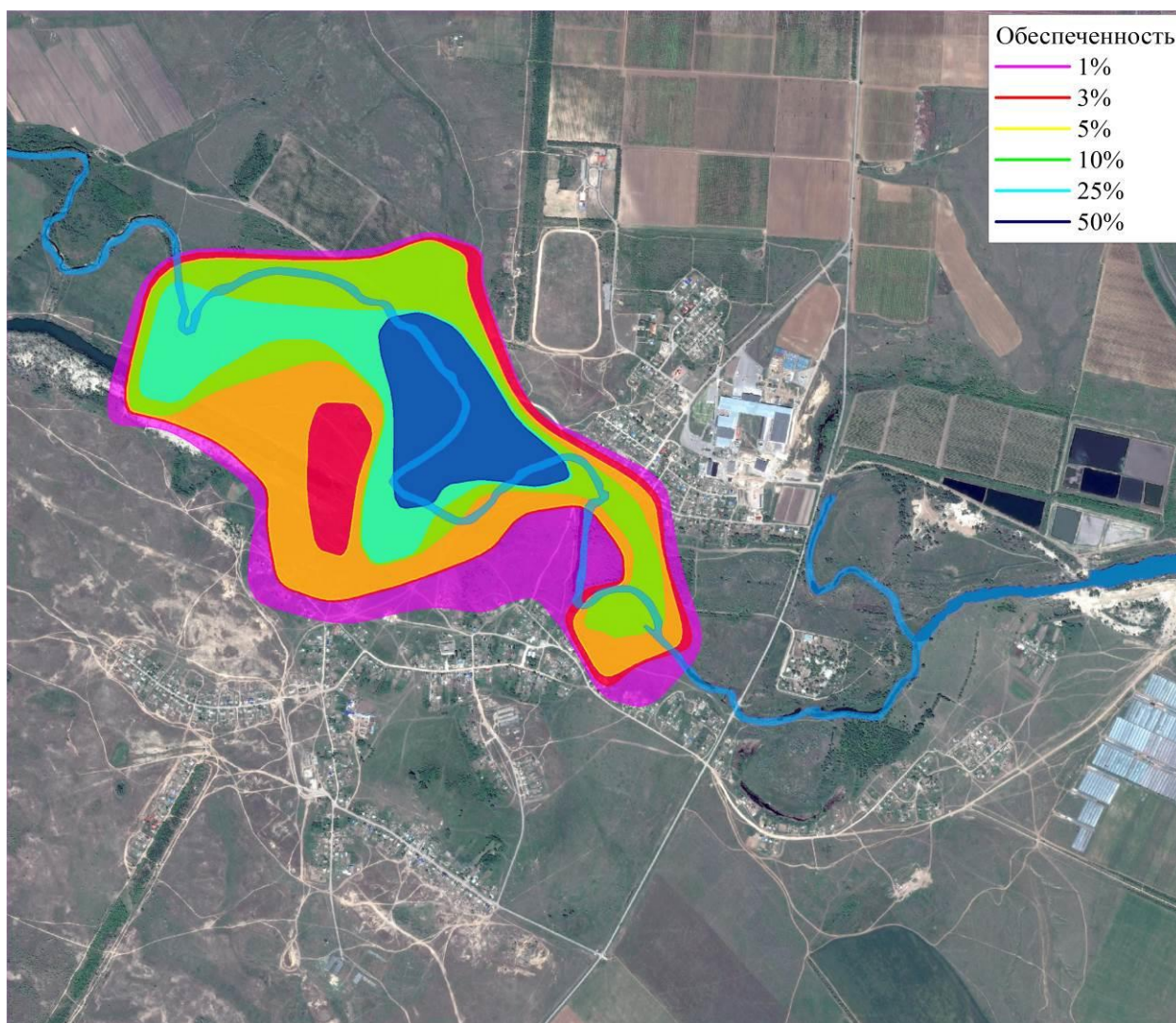
Рис. 8: Границы зон затопления в окрестности х. Паньшино при различной обеспеченности на космическом снимке. Сплошные линии соответствуют границам с глубиной 0.1 м, полупрозрачная цветная заливка соответствует зонам затопления заданной обеспеченности.
