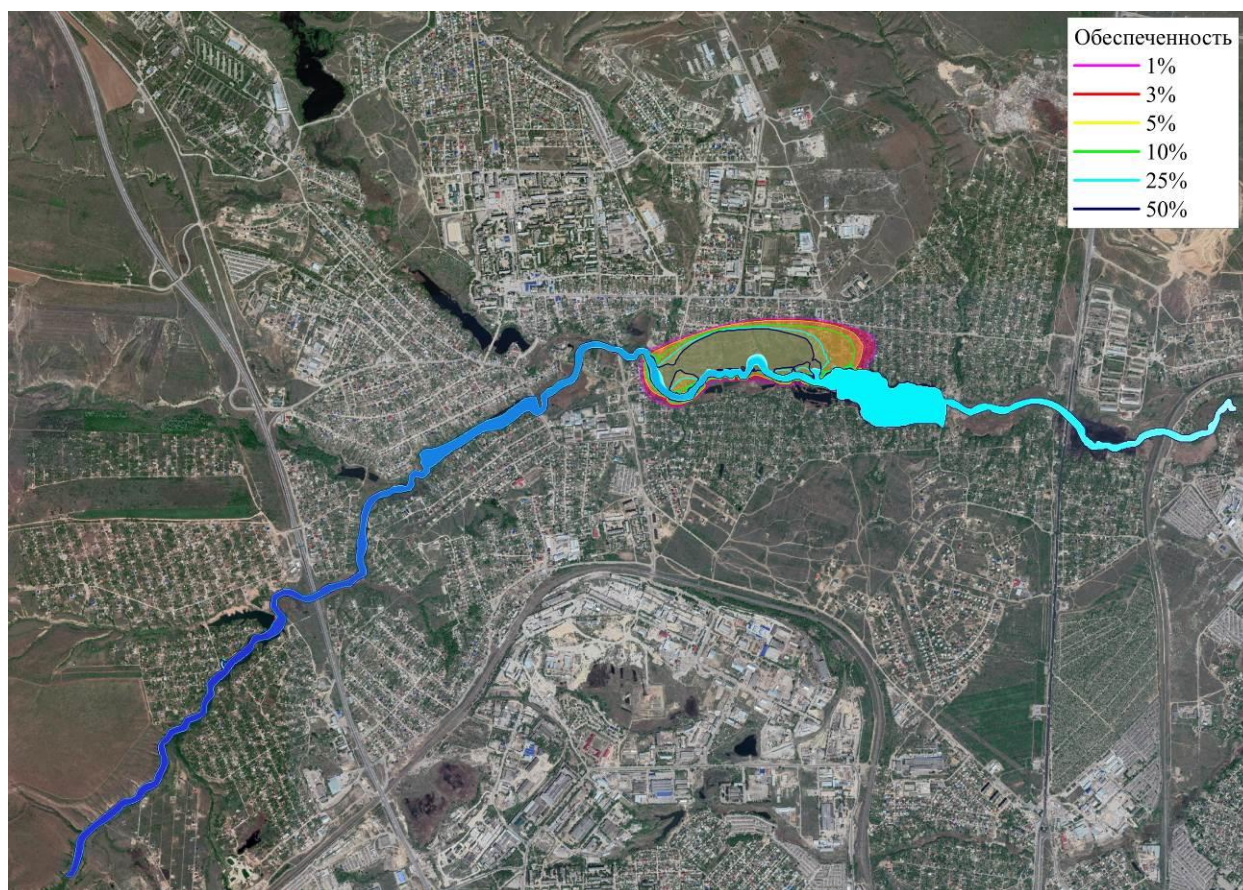
Рис. 7: Границы зон затопления в окрестности р.п. Городище при различной обеспеченности на космическом снимке. Сплошные линии соответствуют границам с глубиной 0.1 м, полупрозрачная цветная заливка соответствует зонам затопления заданной обеспеченности.
